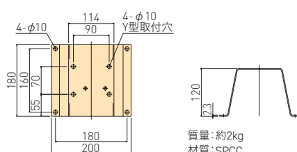
PS-X:CM-Y用(塗装色:マンセル7.5GY 5/4.5)
