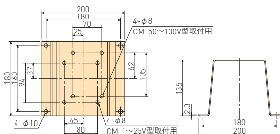
PS-V:CM-V用(塗装色:マンセル7.5GY 5/4.5)
