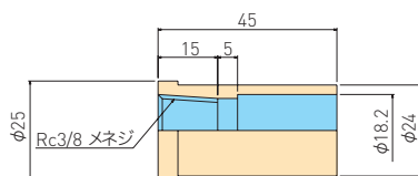
型 式:SW-3 (Rc-3/8×VP13A)
