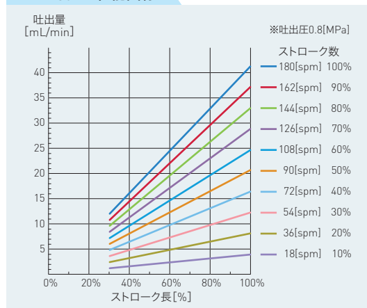
MP-L30P 性能曲線
