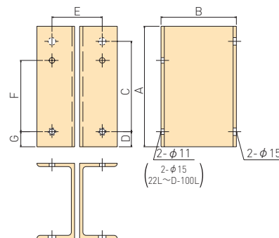
PS-G・L1~L2:CM-G・R・L用 (塗装色:(PS-G)マンセル2.5PB 5/2、(PS-L1~L3)マンセル2.5PB 2.5/7)
